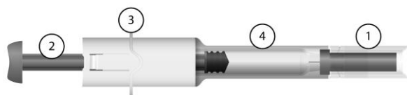
Figura 1. Seringă cu sistem automat de protecție
